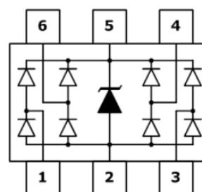
SOT-363
