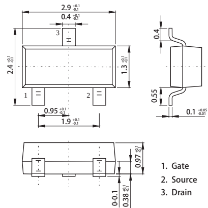
SOT-23
