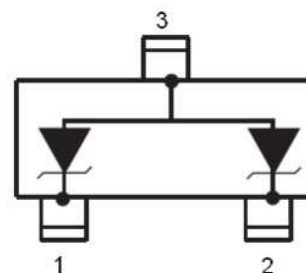
SOT-23
