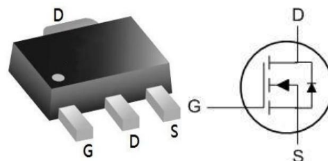
SOT89-3L
