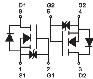
SOT-563
