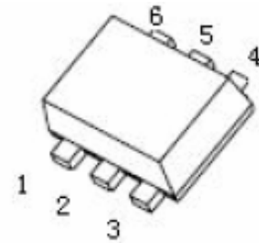
SOT-563
