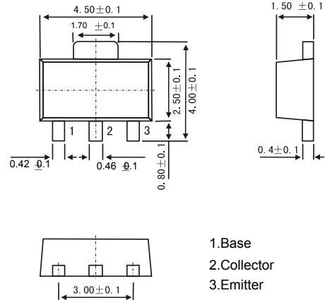
SOT-89
