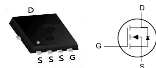
PDFN5060-8L
