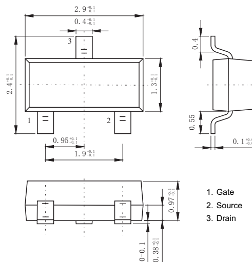
SOT-23
