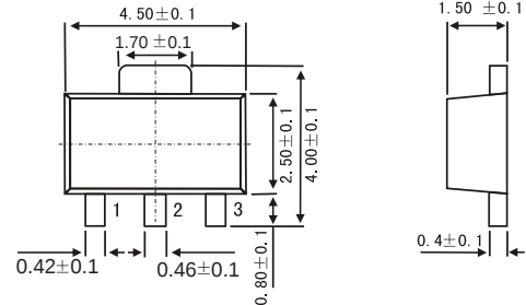
SOT-89
