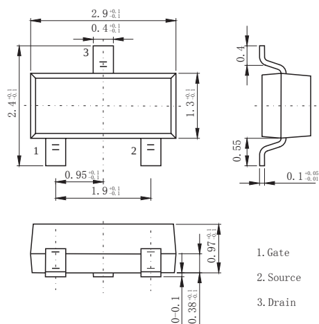
SOT-23
