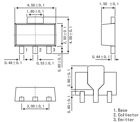
SOT-89
