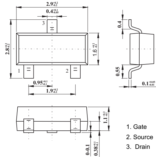
SOT-23-3
