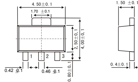
SOT-89
